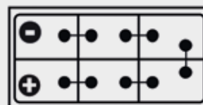
SCHALTUNG 4
