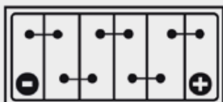
SCHALTUNG 0
